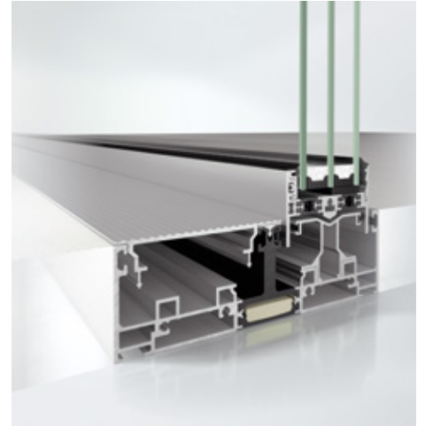
Prag la nivelul podelei și toc de 57 mm Level threshold in 57 mm outer frame
