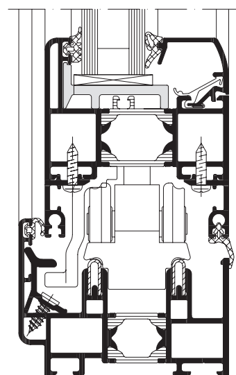
Schüco ASS 70 FD, scara 1:2 Schüco ASS 70 FD, scale 1:2
