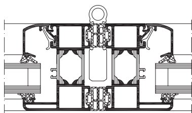
Schüco ASS 70 FD, scara 1:3 Schüco ASS 70 FD, scale 1:3
