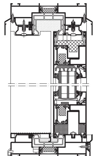
Schüco ASS 70.HI, scara 1:5 Schüco ASS 70.HI, scale 1:5
