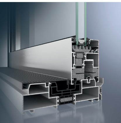
Sistem glisant cu ridicare Schüco ASS 70.HI Schüco lift-and-slide system ASS 70.HI
